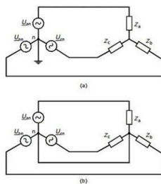
Fig.3.6 Sistem e lidhura në yll me tre dhe katër përçueshës (a) sistemi me tre përçueshës (b) sistemi me katër përçueshës
